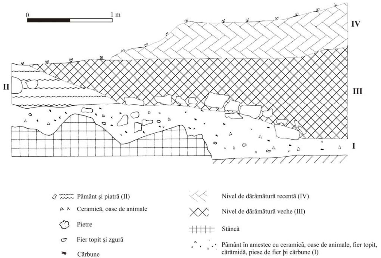
Fig. 1. Carașova. Profilul nordic al S5/2001.
