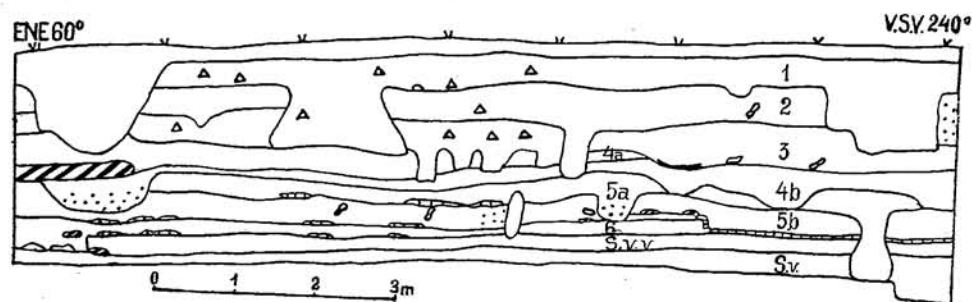
Fig. 4. — Stoicani-Cetățuie 1948. Profilul peretelui de Sud al șanțului B.
